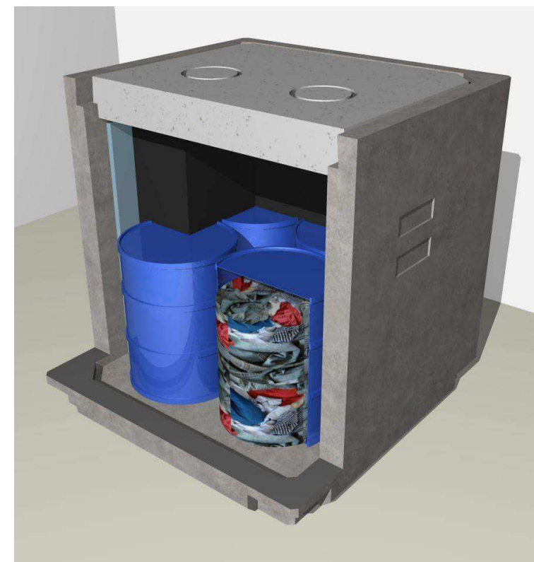
zaplnený vláknobetónový kontajner
